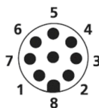
M12 A-coded 8-конкт. "мама"
